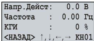
Рисунок 6.13 – Экран измеряемых значений для канала 1
