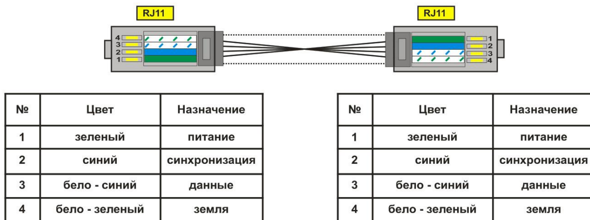
Рисунок 5.2 – Нумерация выводов кабеля КМР-11-1
