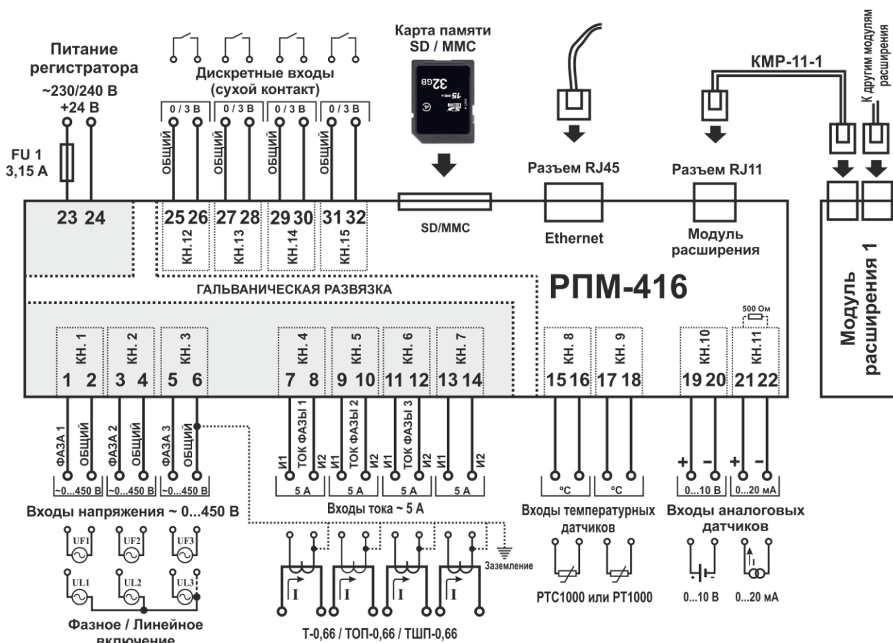
FU1 – Предохранитель (автоматический выключатель) на ток 3,15 А
