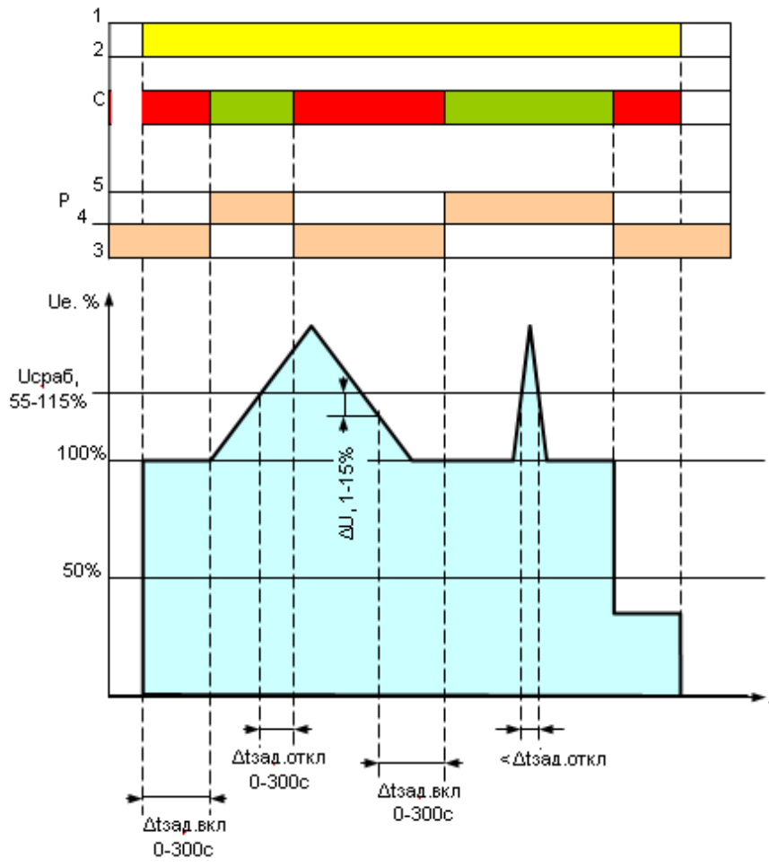
Рисунок 4 - Диаграмма работы реле НЛ-18-1
